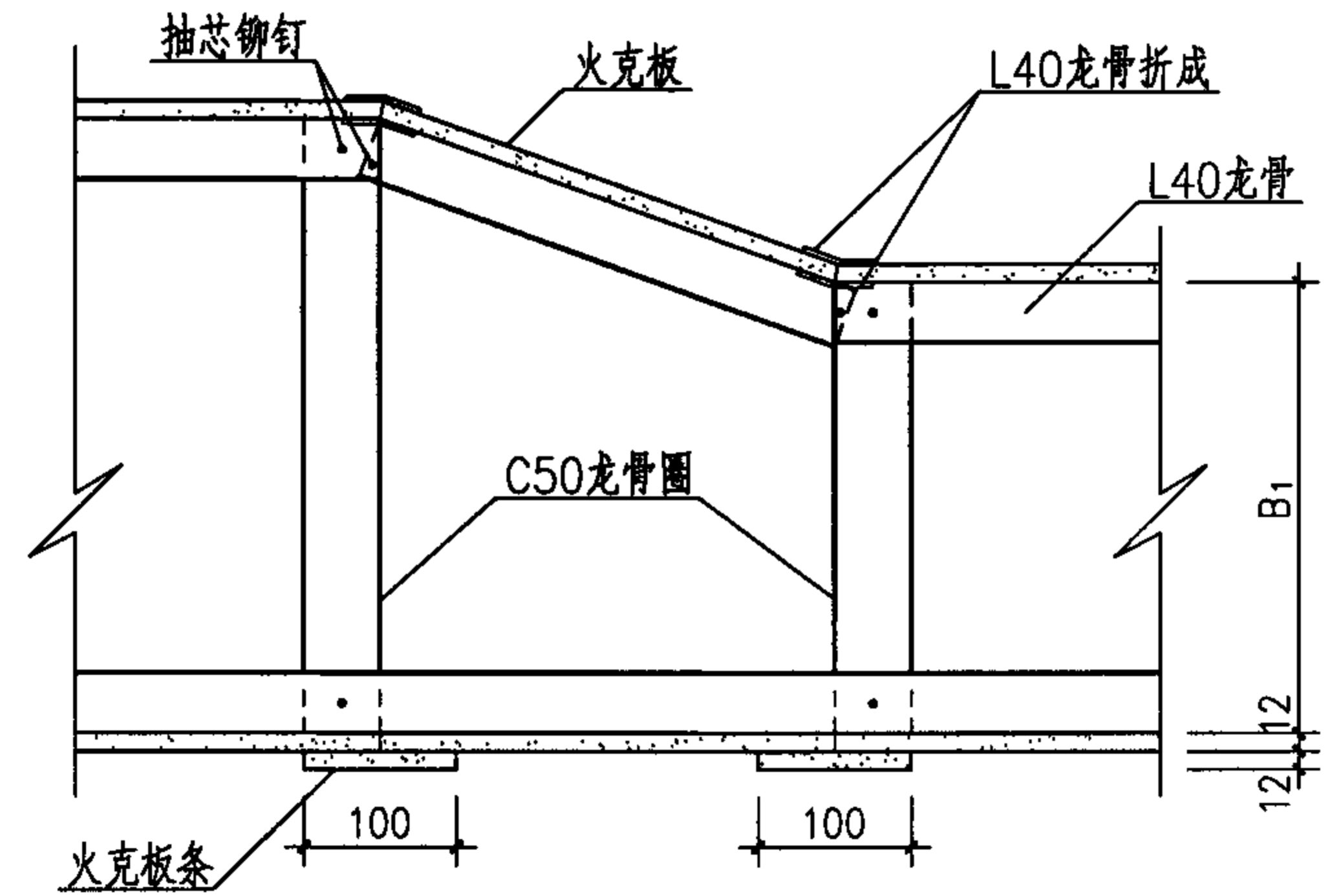
变径
