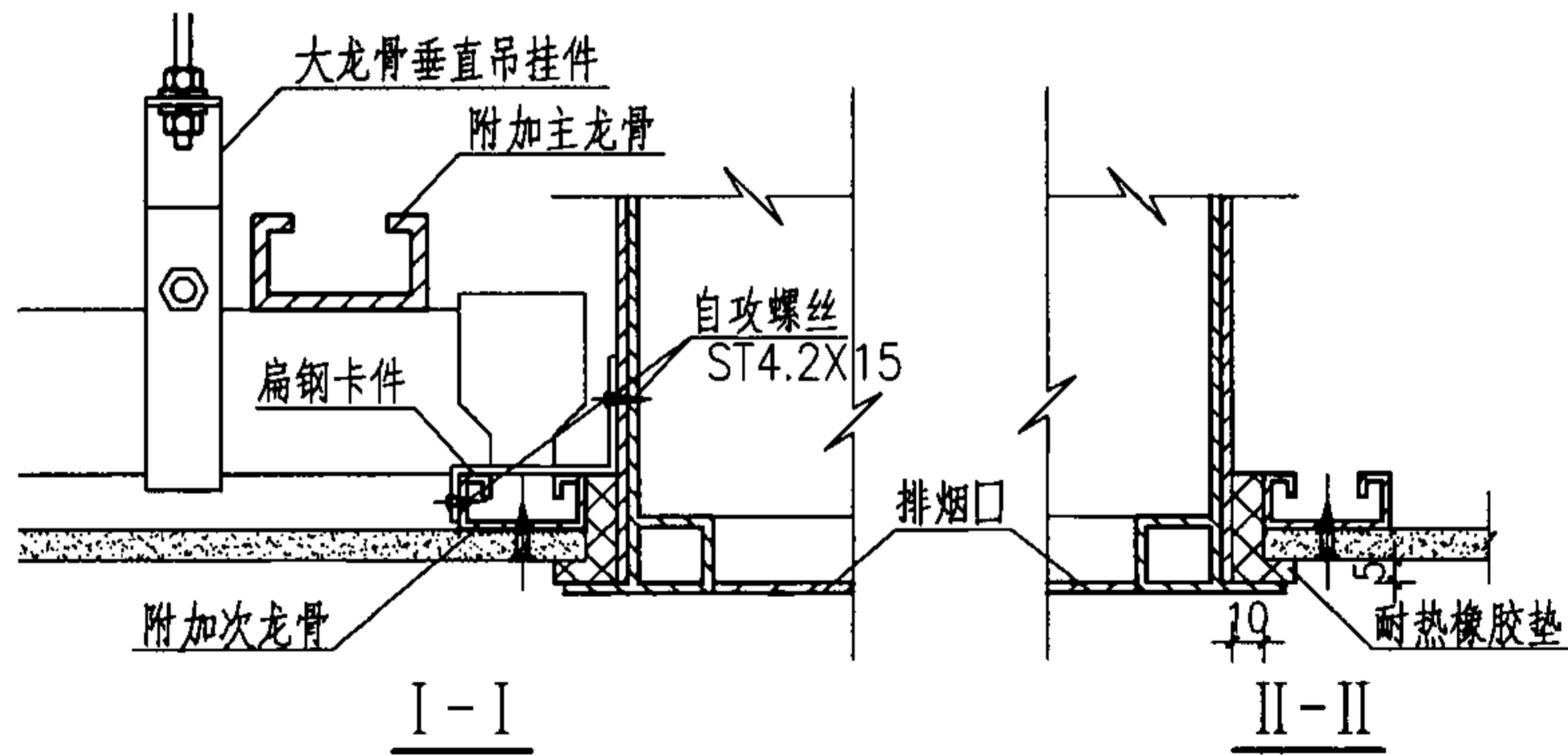
吊项龙骨详图
