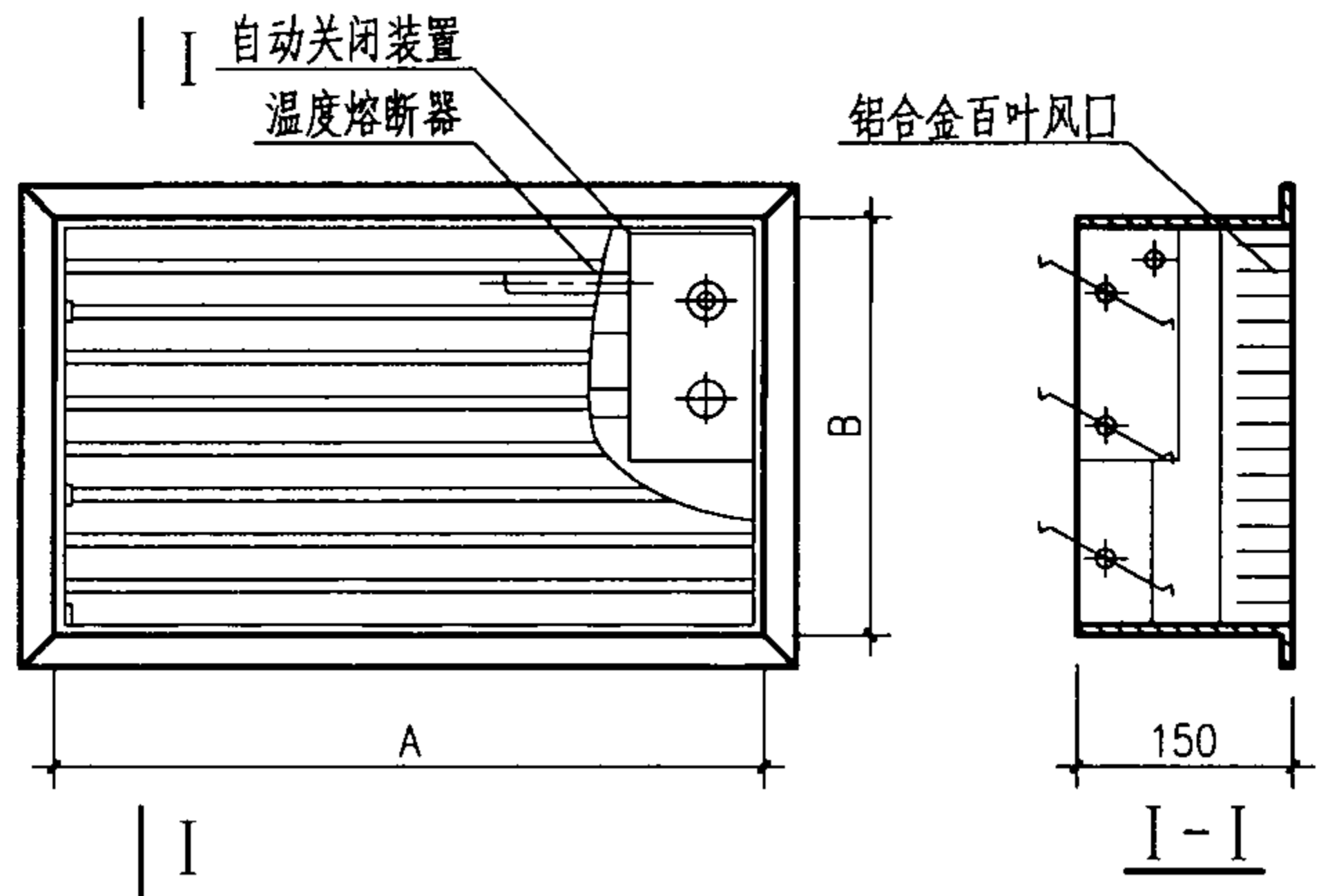
防火风口
