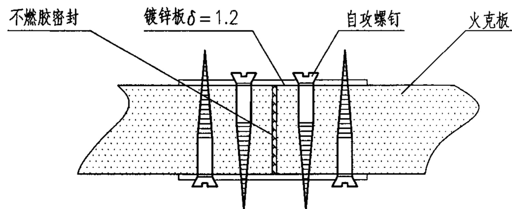
防火风管板材的连接
