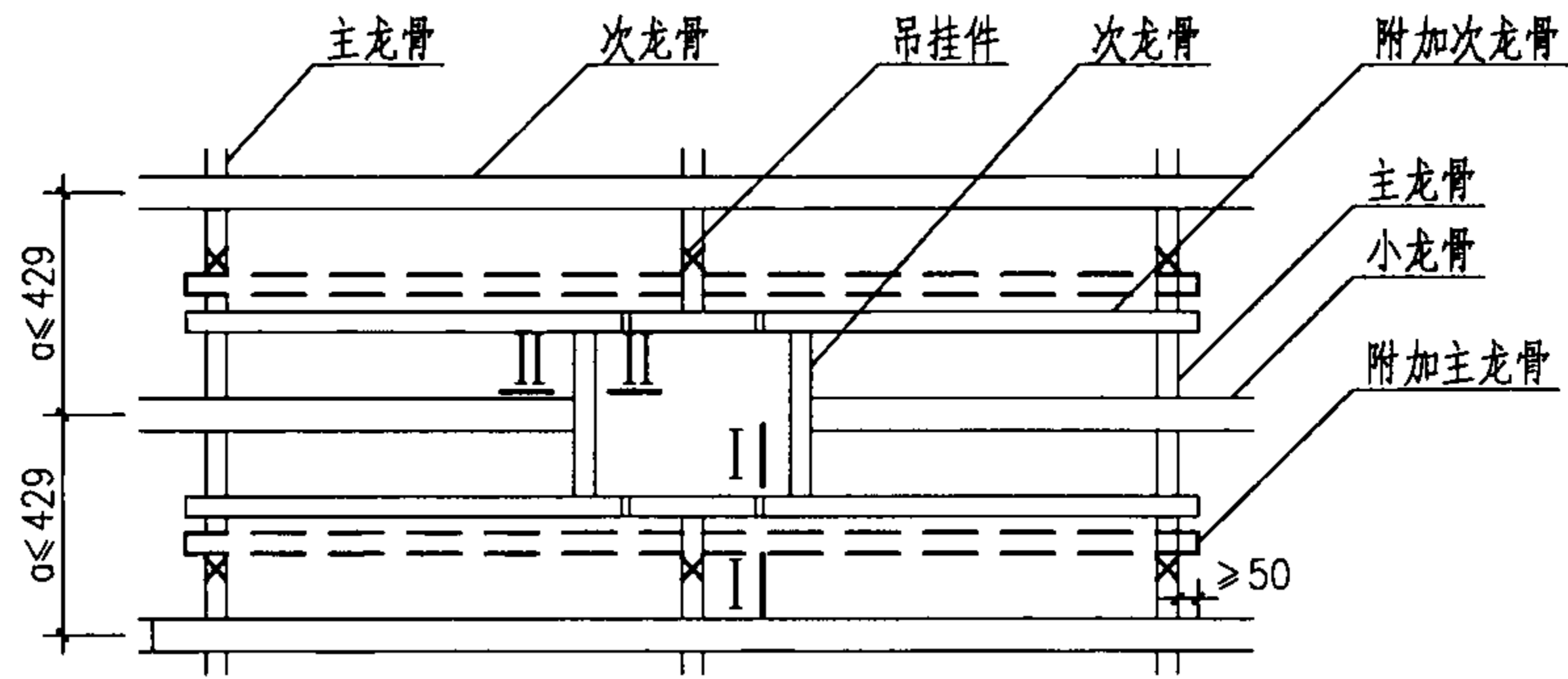
吊项龙骨详图
