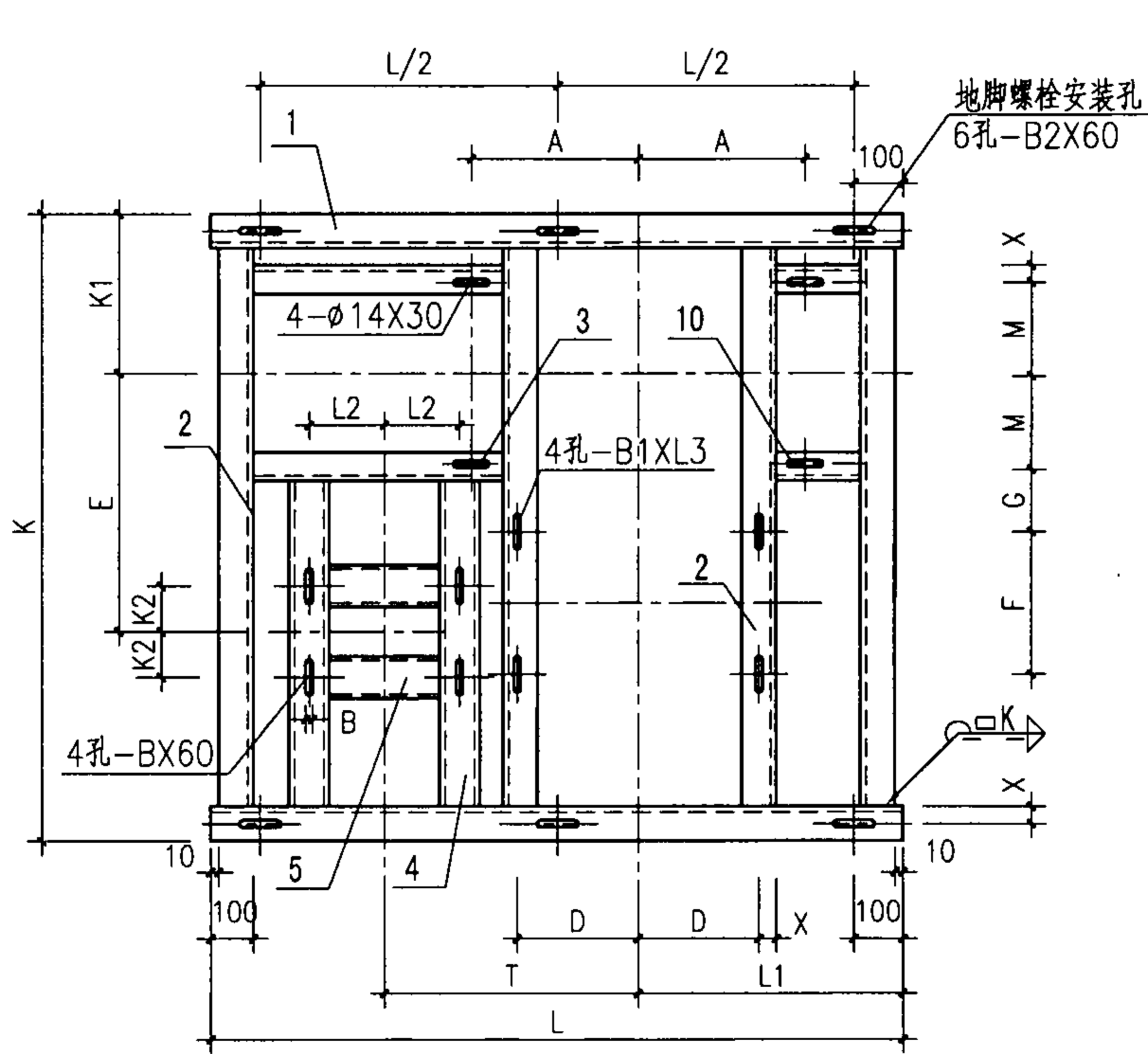
底架详图
