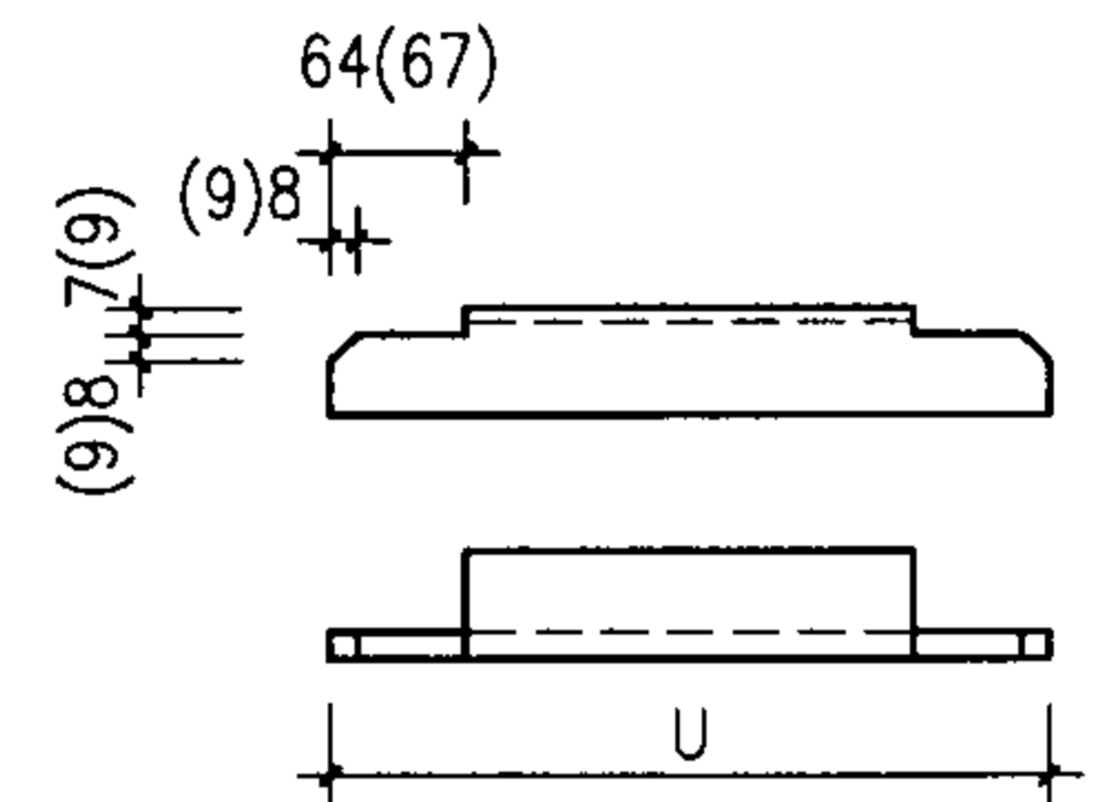
件号7详图
