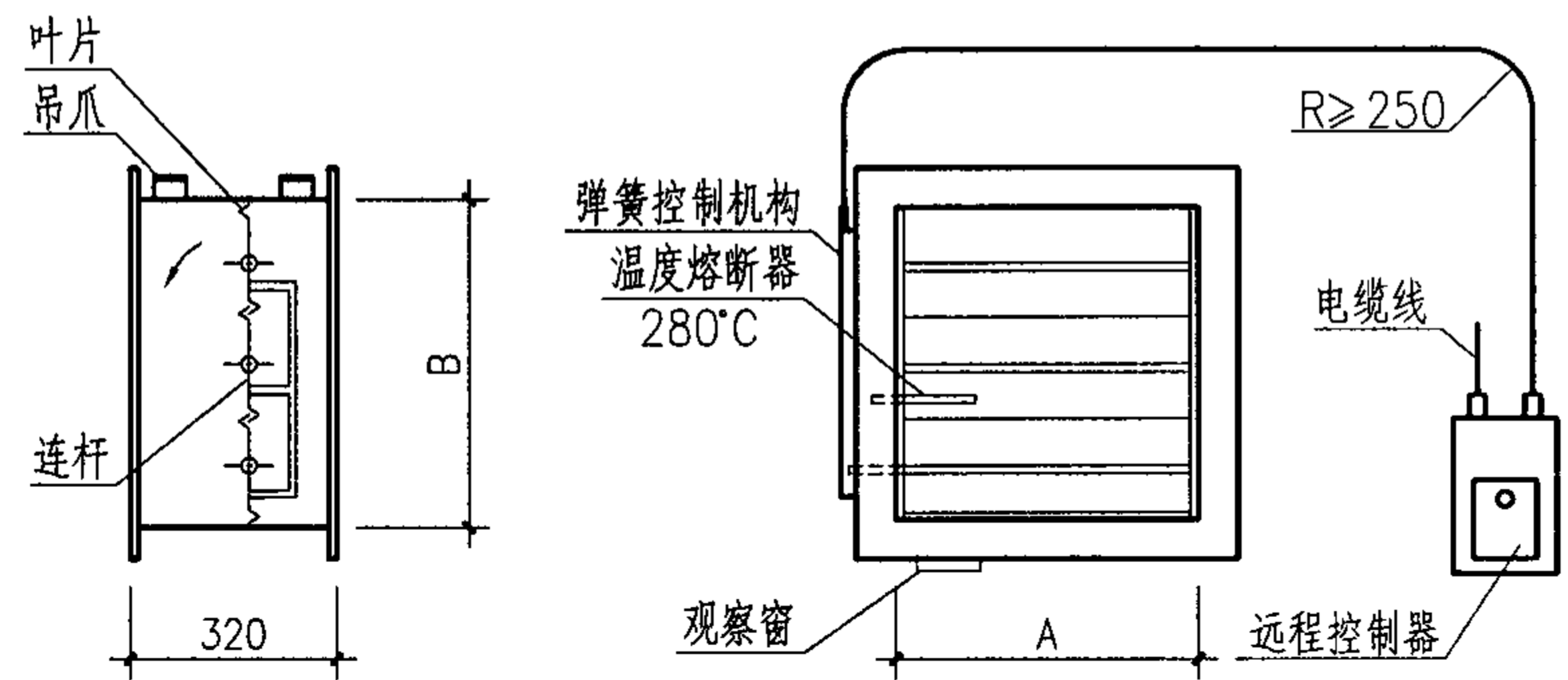
矩形远控排烟防火阀
