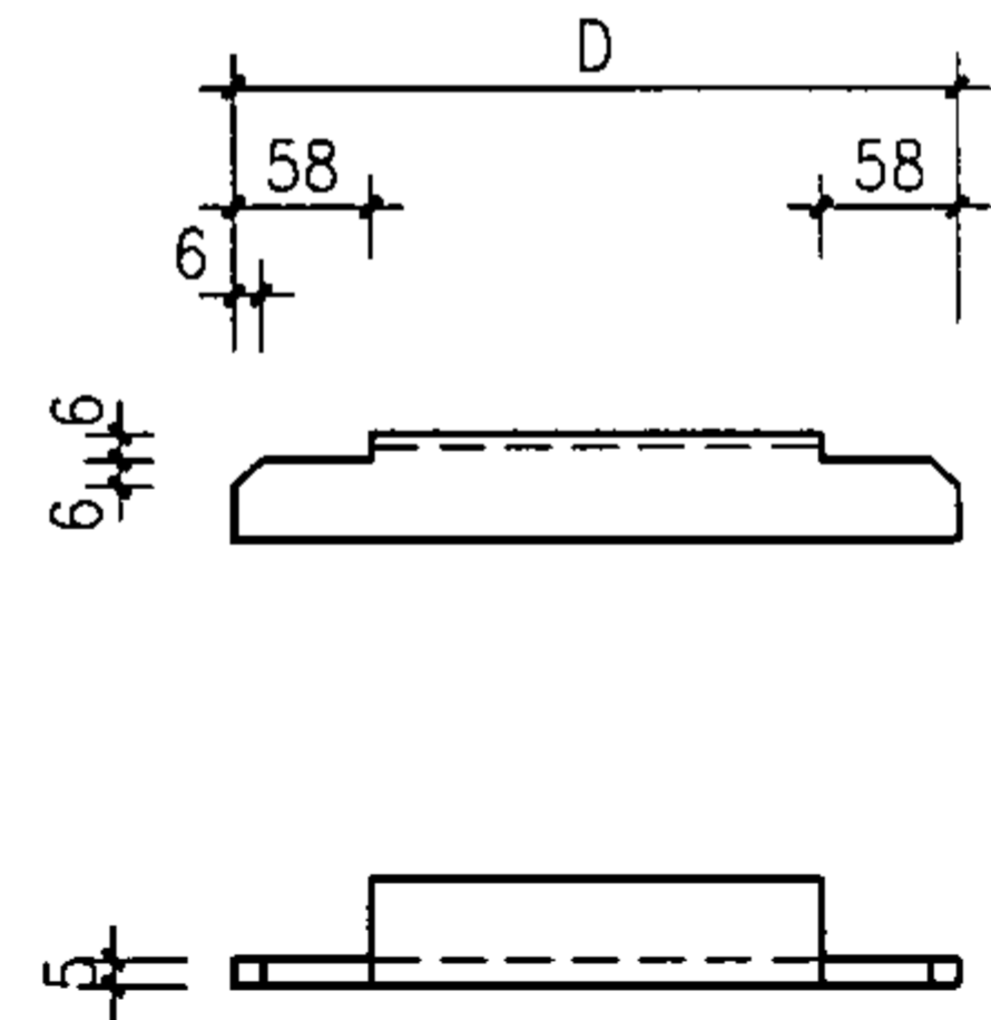
件号4详图
