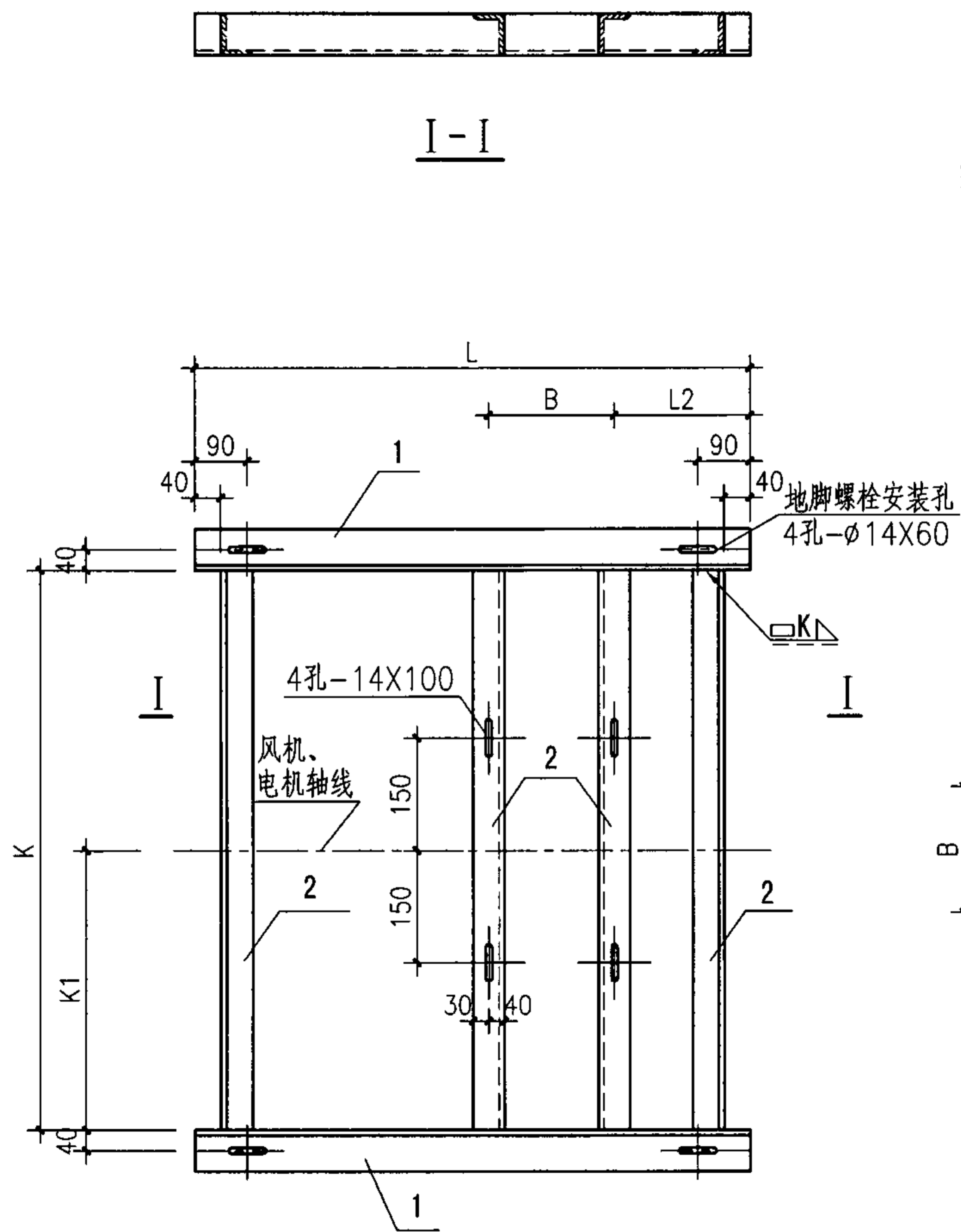
底架详图
