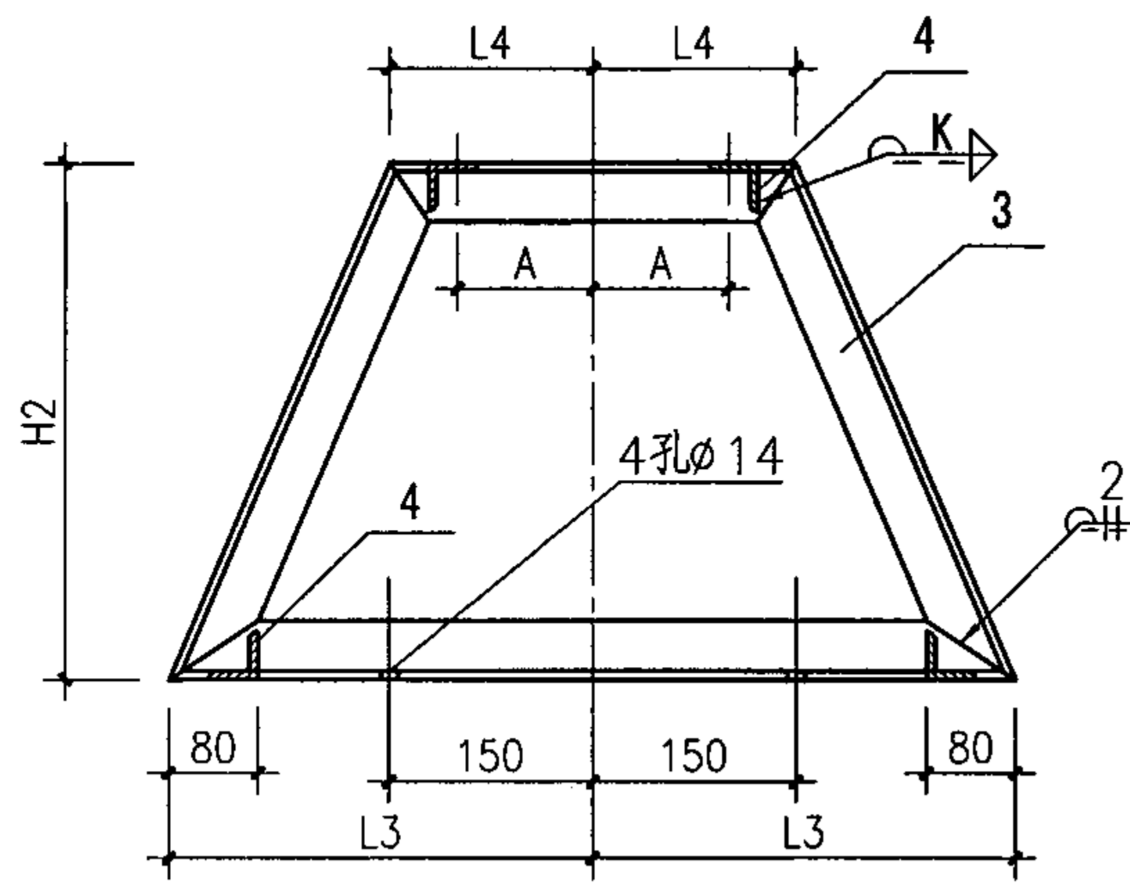
II-II
