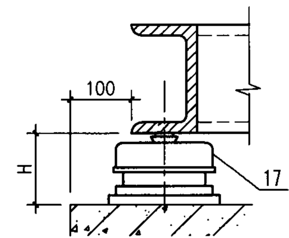
① 弹簧减振器安装
