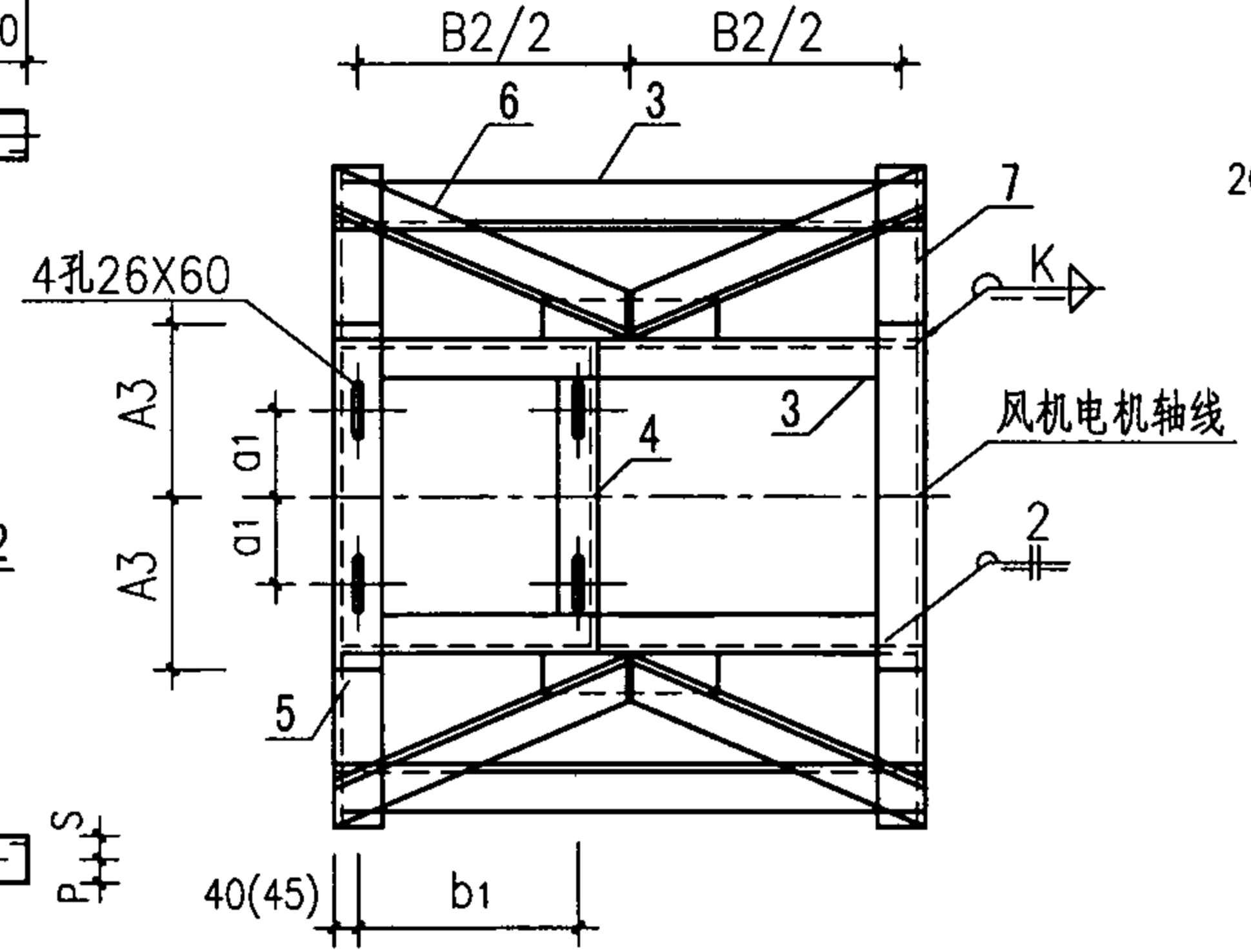
轴承箱及电机支座详图
