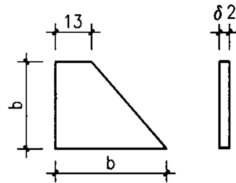
件号2
