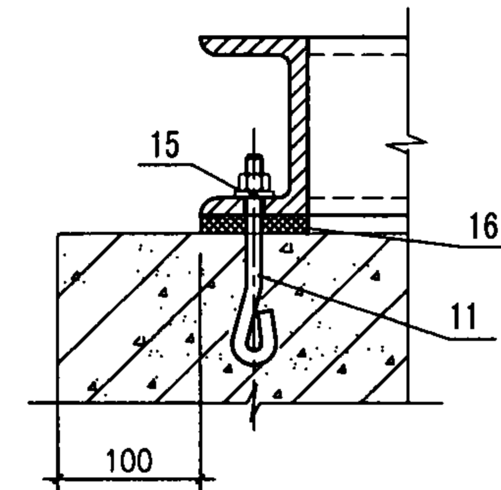
① 地脚螺栓安装
