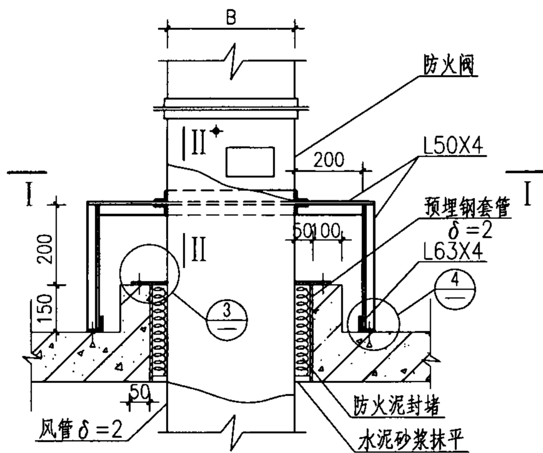
防火阀楼板上安装
