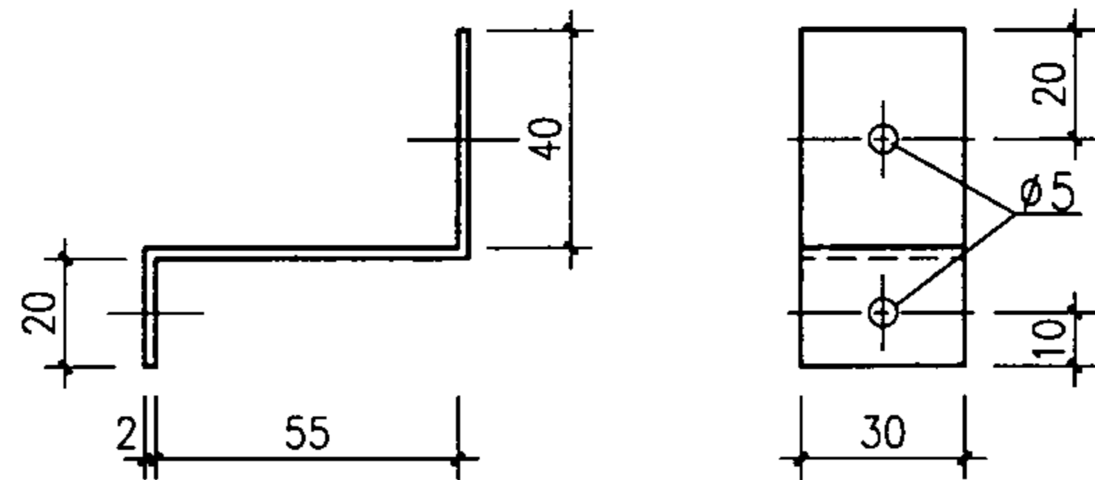
扁钢卡件
