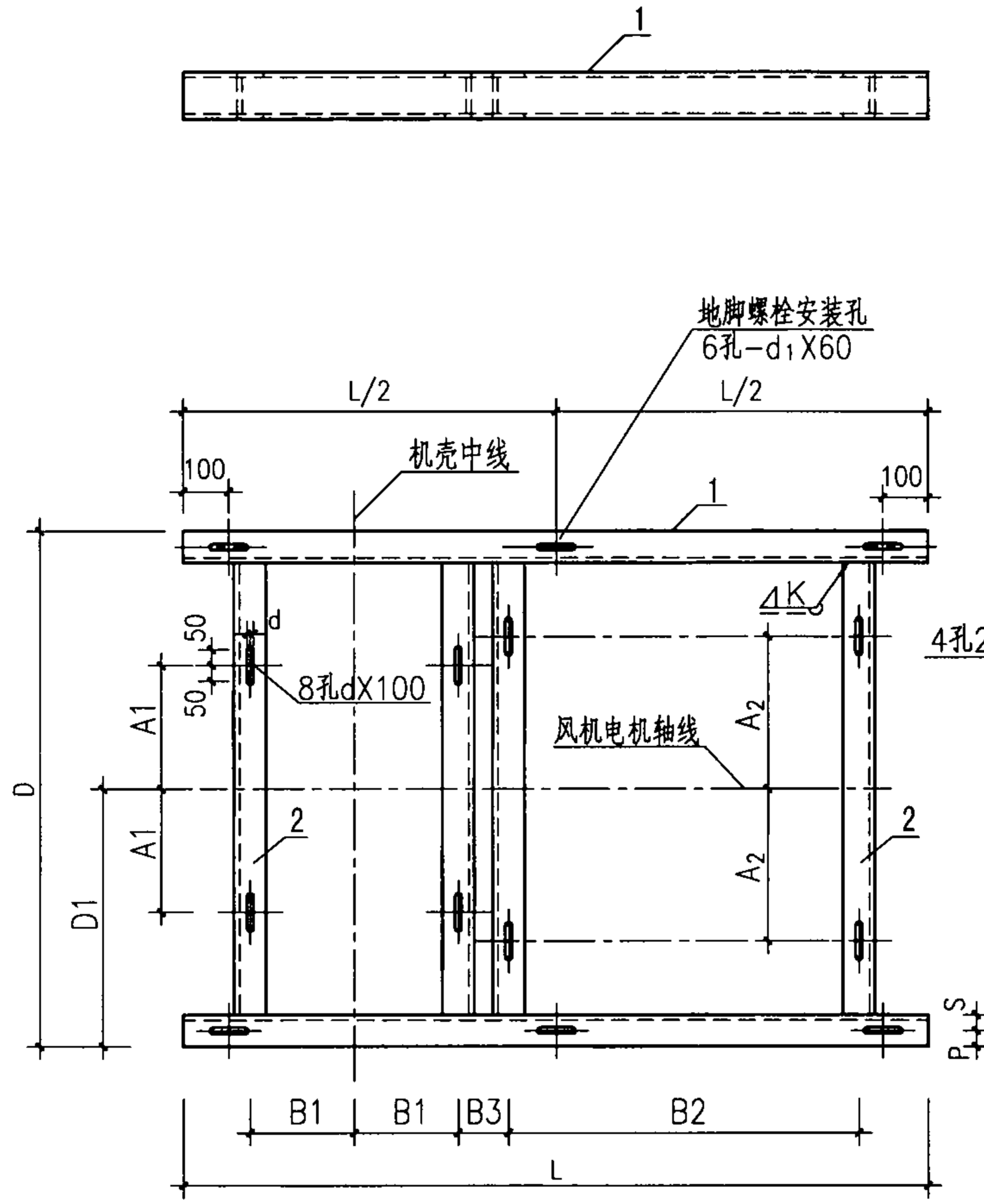
底架详图
