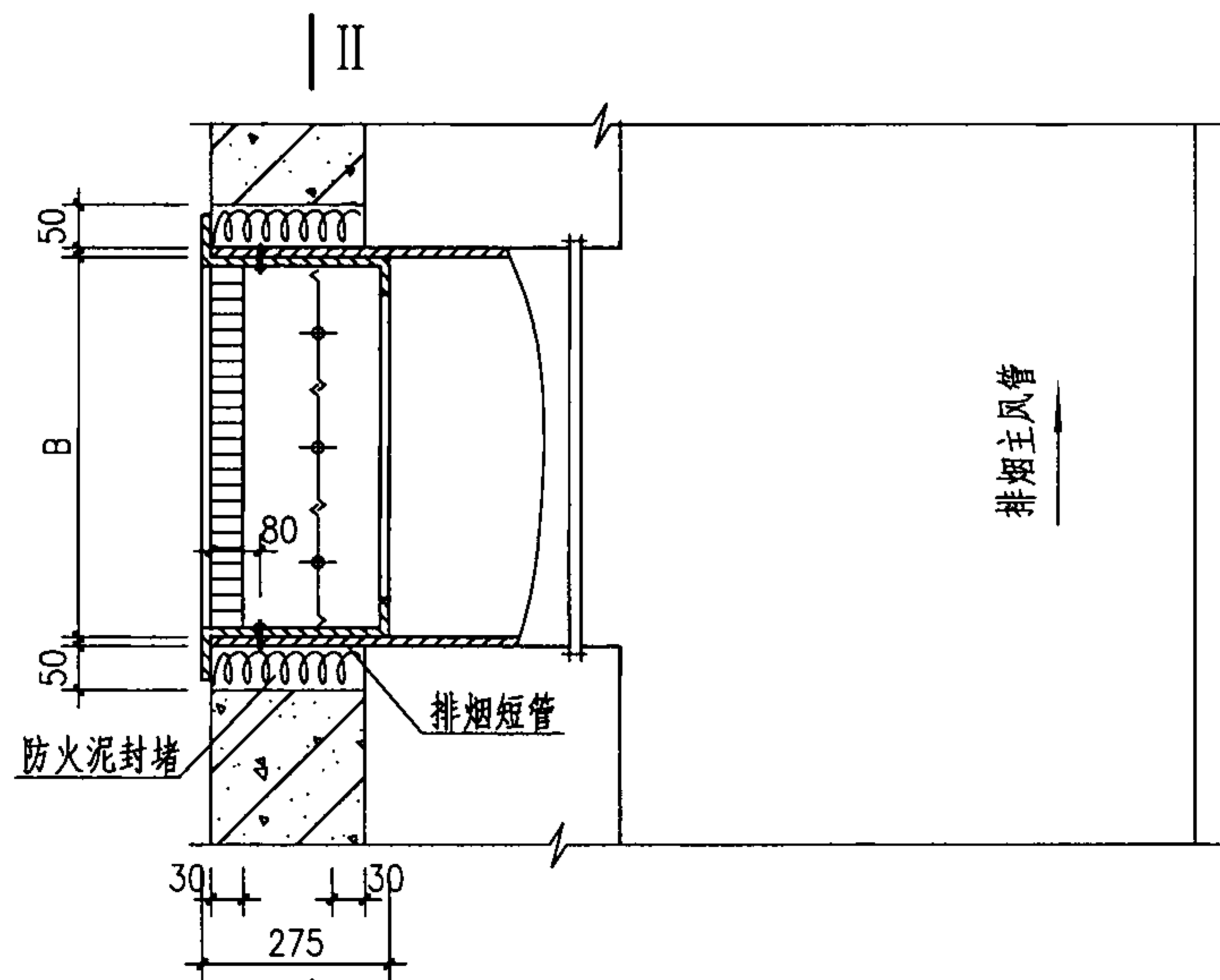
II-II I-I (混凝土墙上安装)
