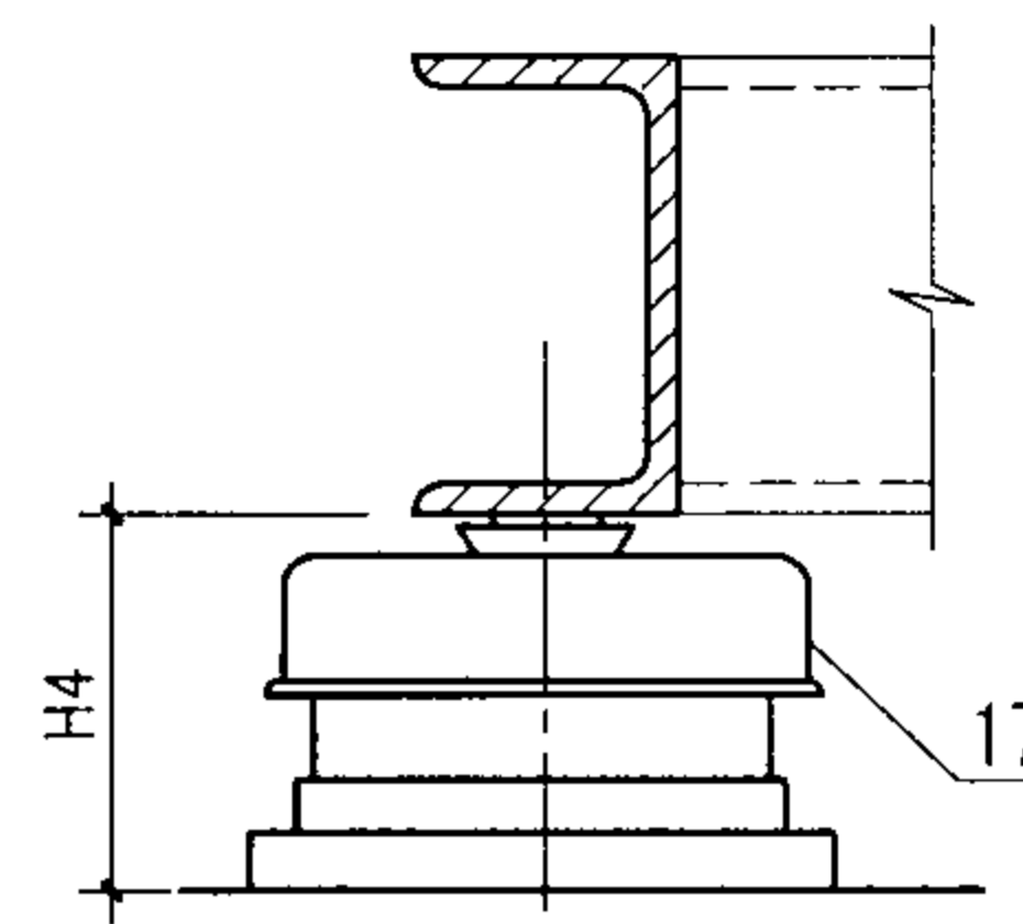
① 弹簧减振器安装
