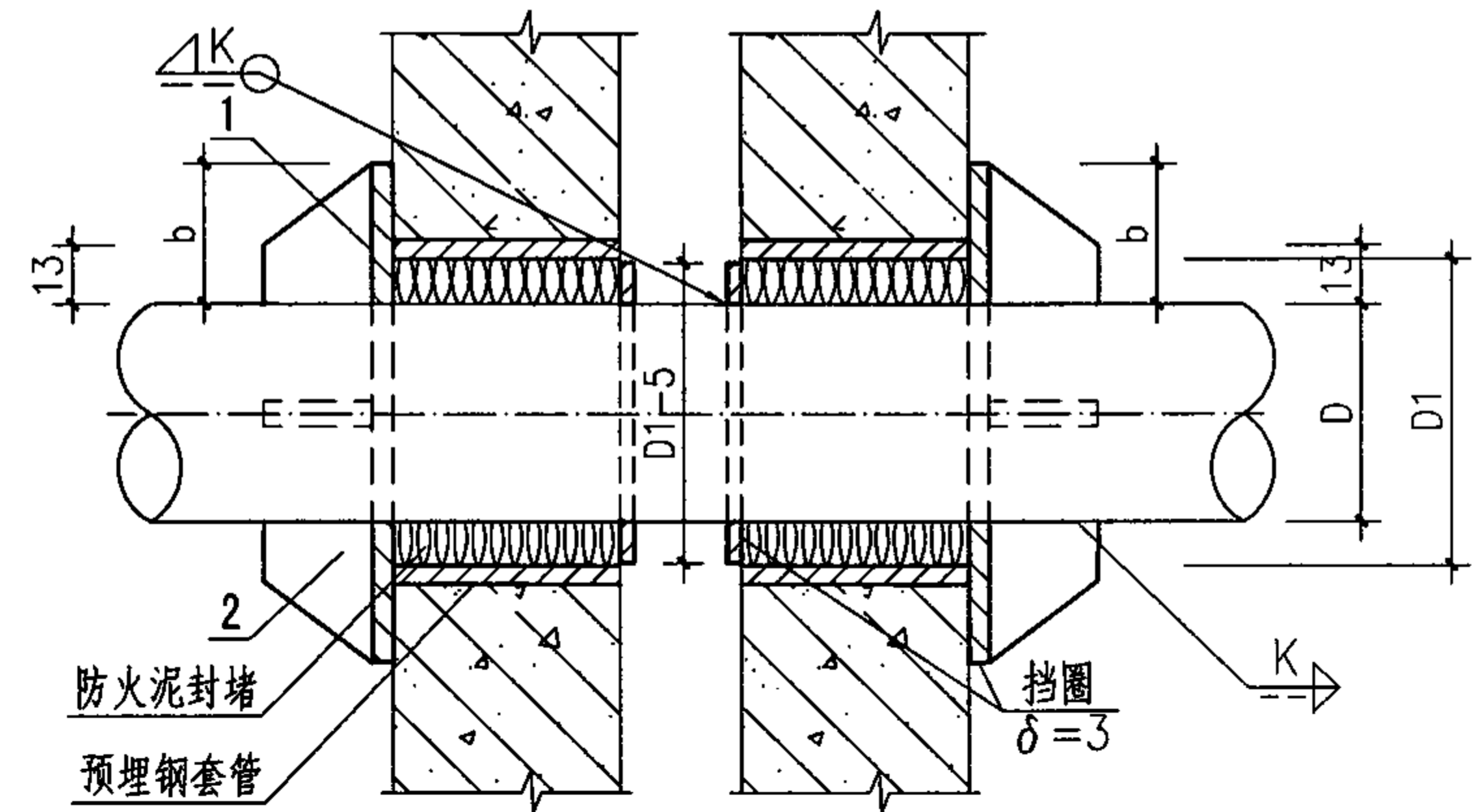
I-I (穿越沉降缝)
